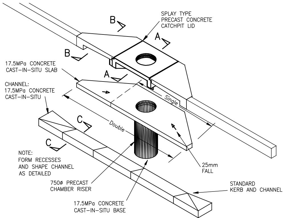
PERSPECTIVE VIEW N.T.S.
